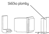
Šroub plomby 16.10.0011.8
